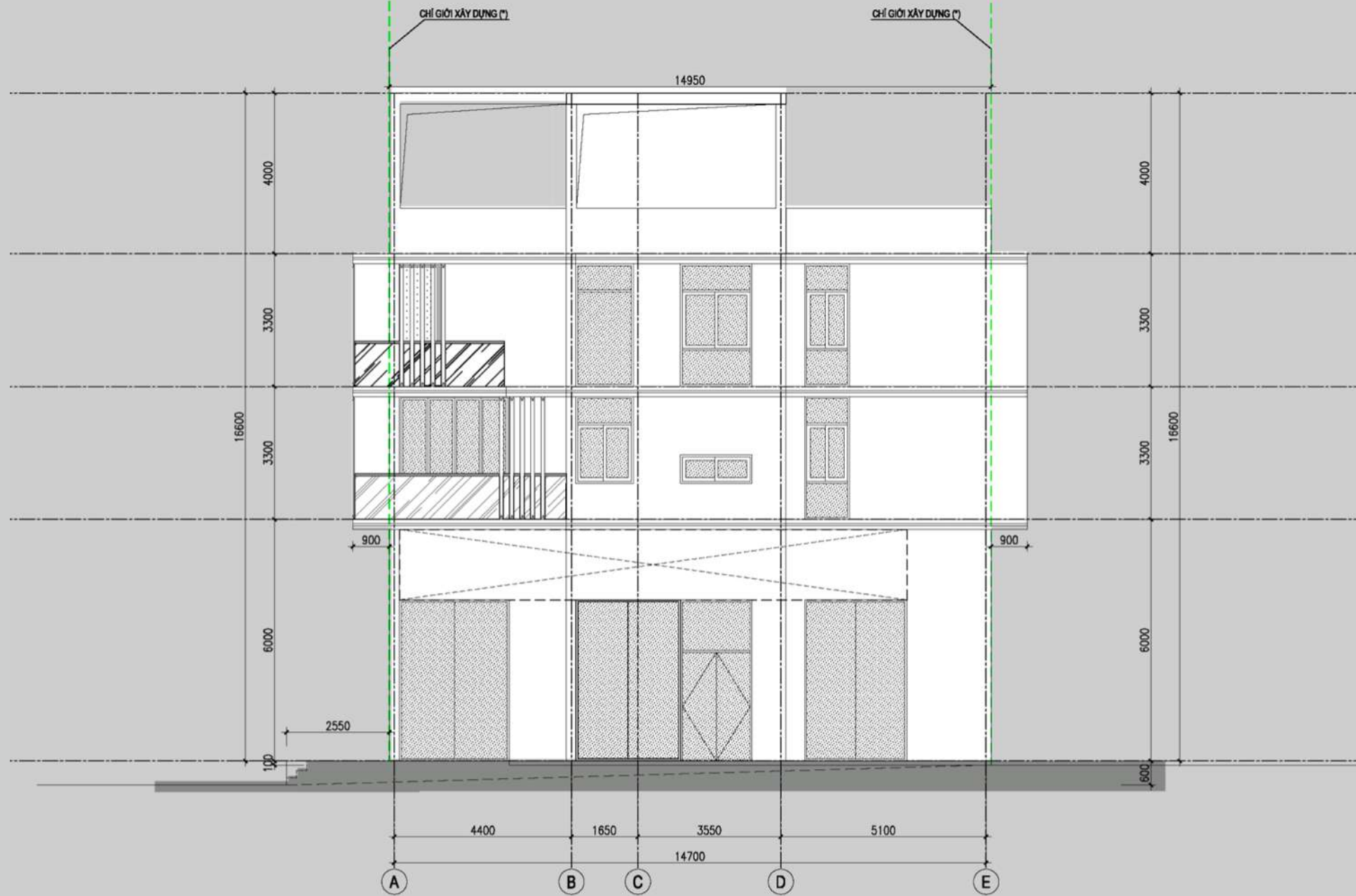
MẶT ĐỨNG A-E
