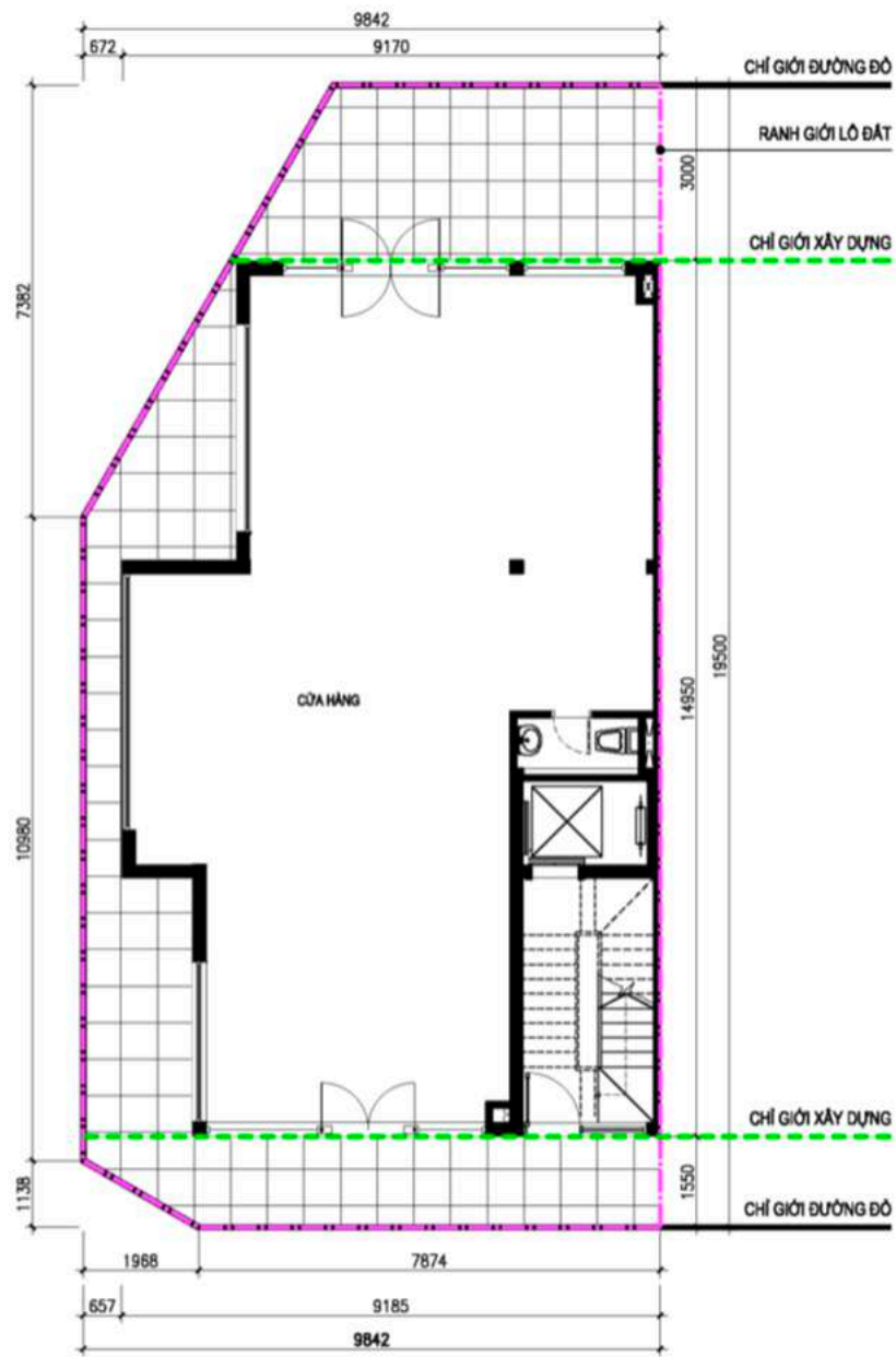
TỔNG MẶT BẰNG BỐ TRÍ MẪU
