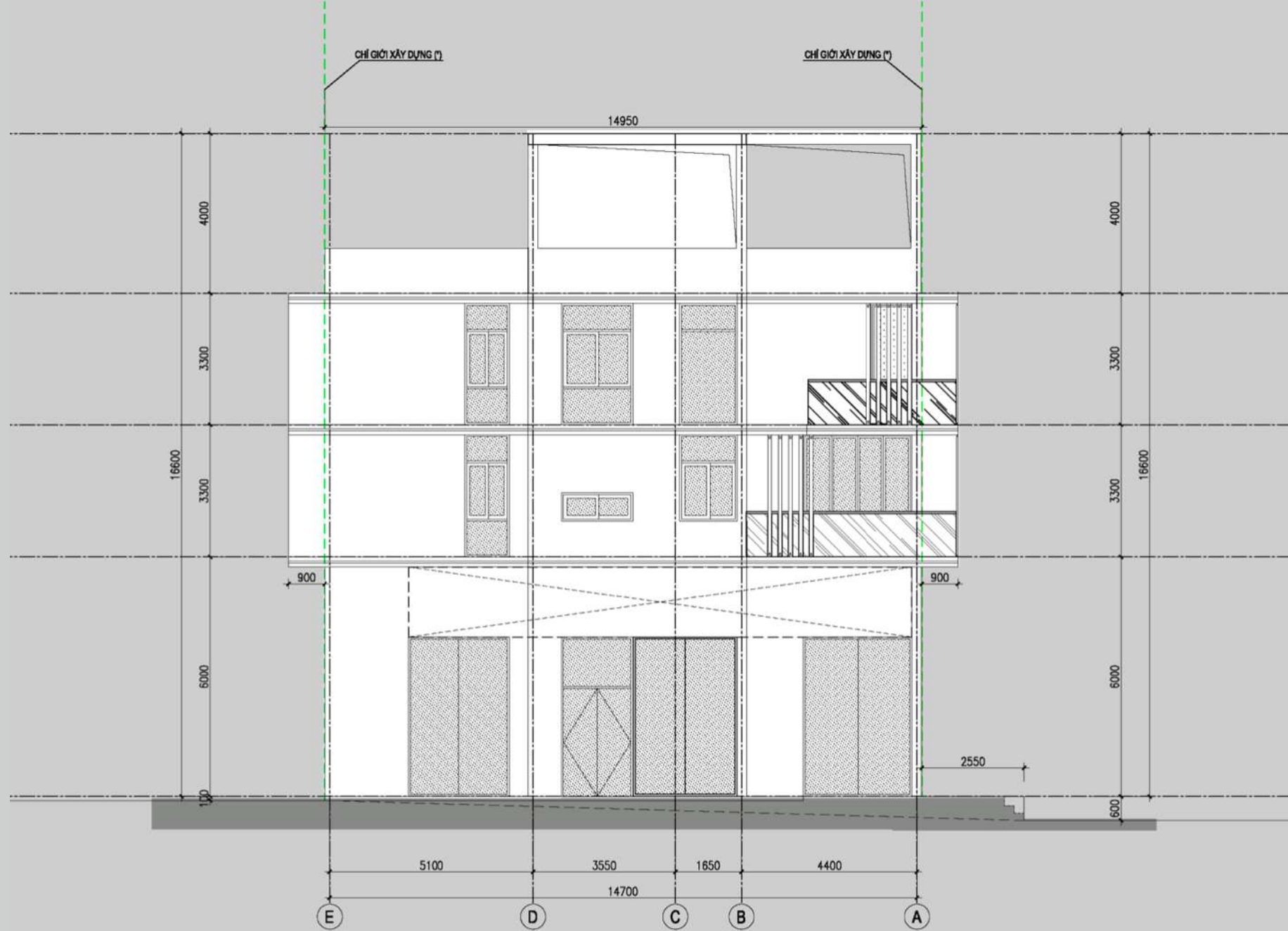
MẶT ĐỨNG E-A
