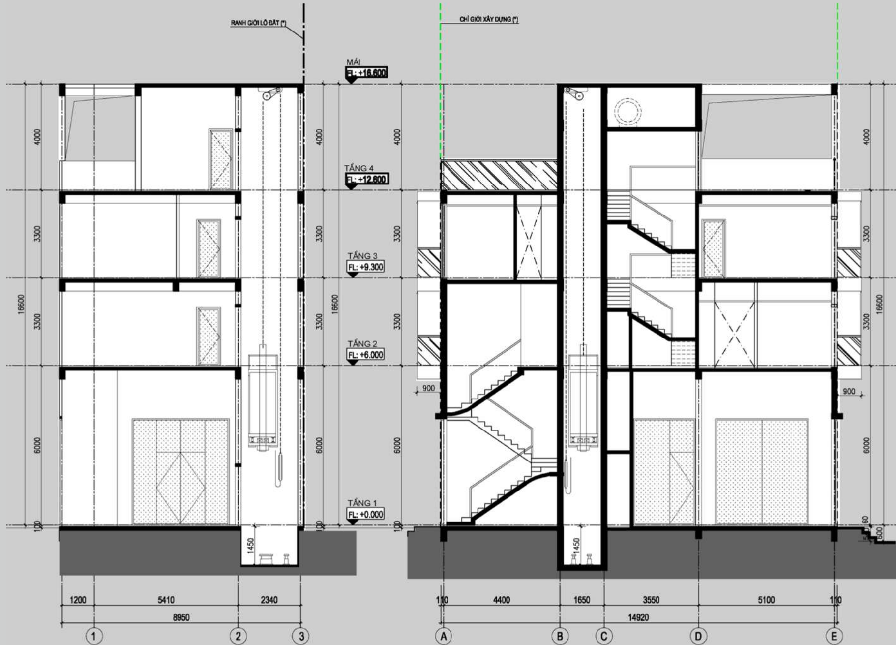
MẶT CẮT NGANG
