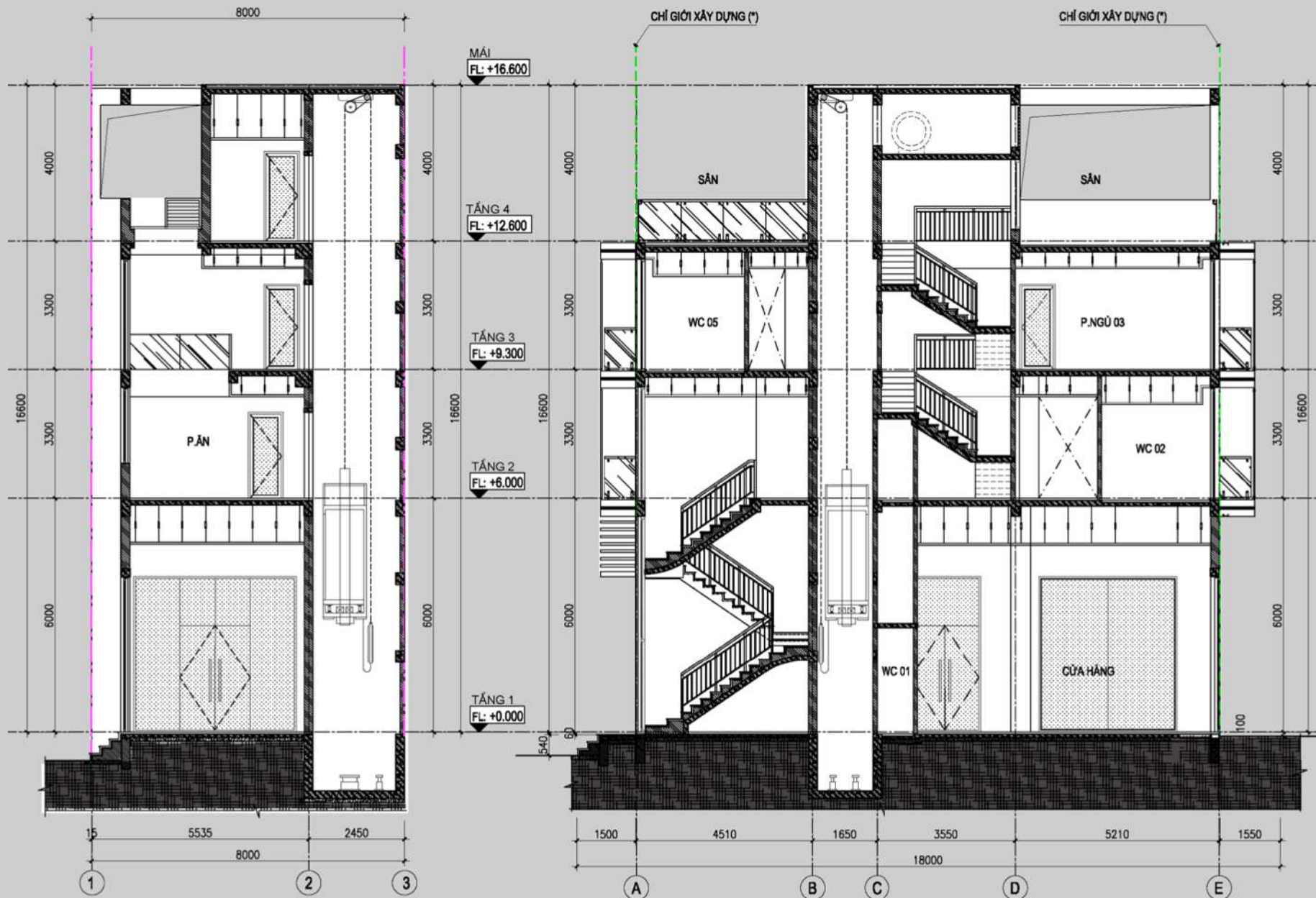
MẶT CẮT NGANG
